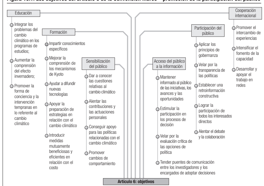
Figura 16.1: Los objetivos del artículo 6 de la Convención Marco – promoción de la participación del público
