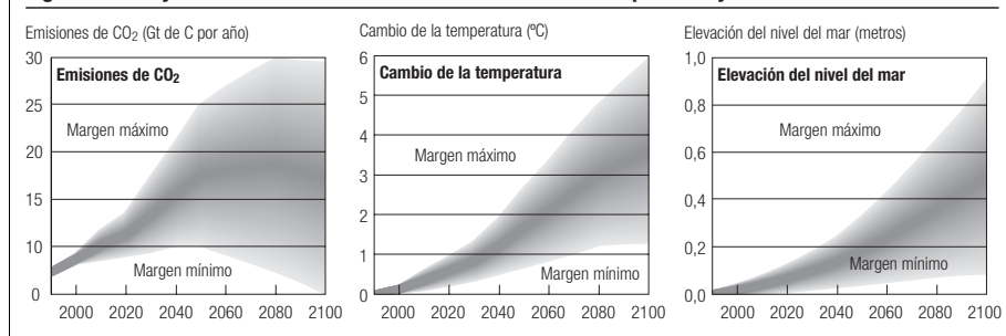
Figura 1.1: Proyección de los efectos de las emisiones sobre temperatura y el nivel del mar
