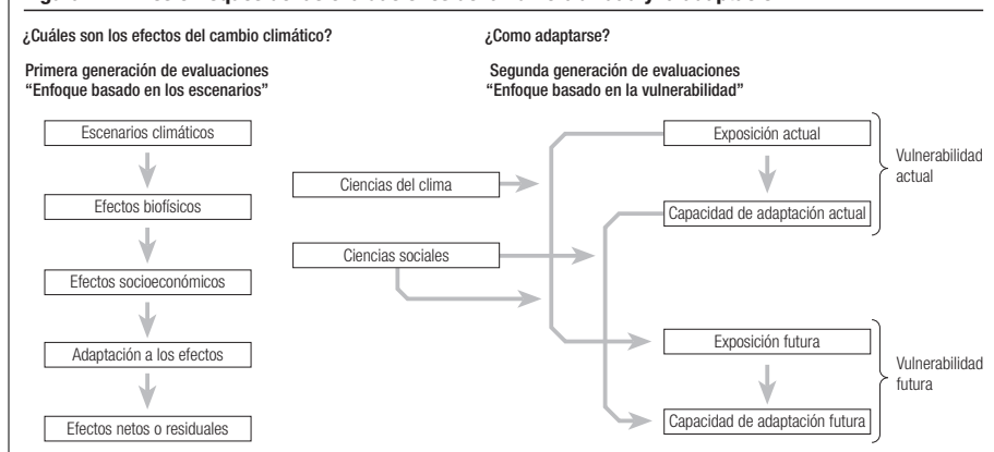
Figura 12.1: Dos enfoques de las evaluaciones de la vulnerabilidad y la adaptación
