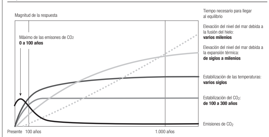
Figura 2: La concentración de CO 2 , la temperatura y el nivel del mar seguirán aumentando hasta mucho después de la reducción de las emisiones
