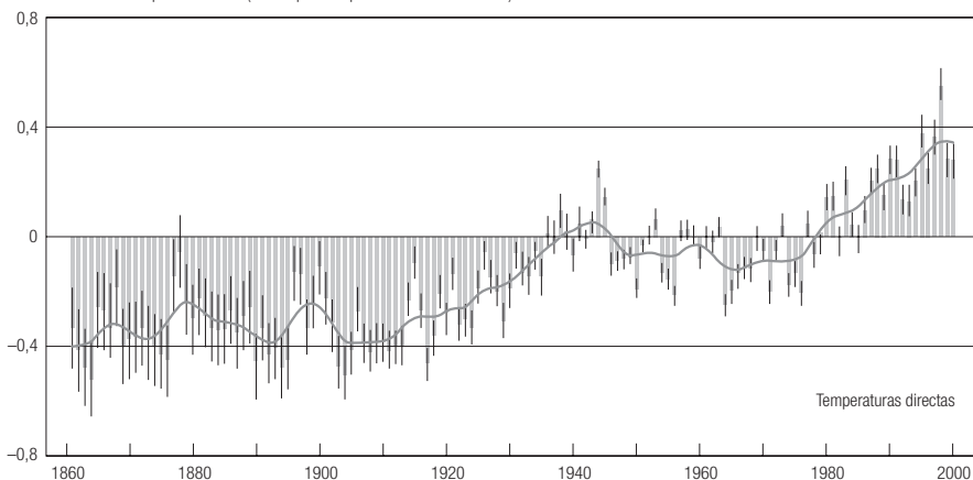
Figura 1: Variación de la temperatura de la superficie de la Tierra en los últimos 140 años
