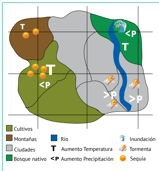
Mapa 4. Municipio de Climatito: amenazas históricas y proyecciones climáticas
