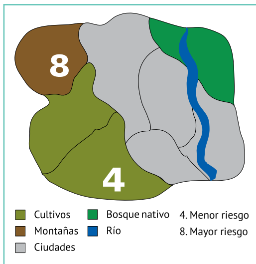
Mapa 8. Municipio de Climatito: estimación del riesgo de sequías, región SO y NO
