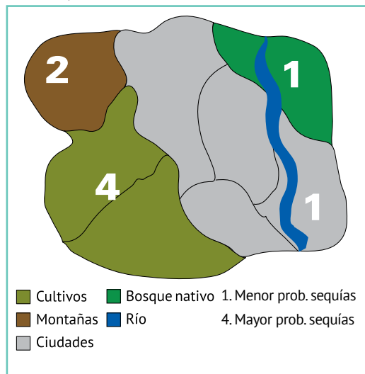
Mapa 5. Municipio de Climatito: probabilidad de ocurrencia de sequías
