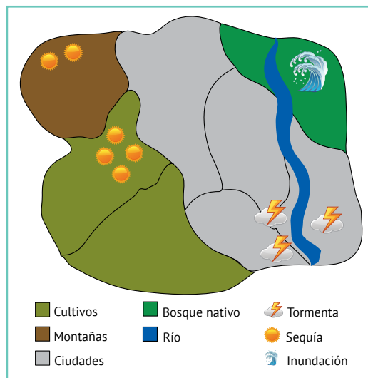
Mapa 2. Municipio de Climatito: amenazas de origen natural
