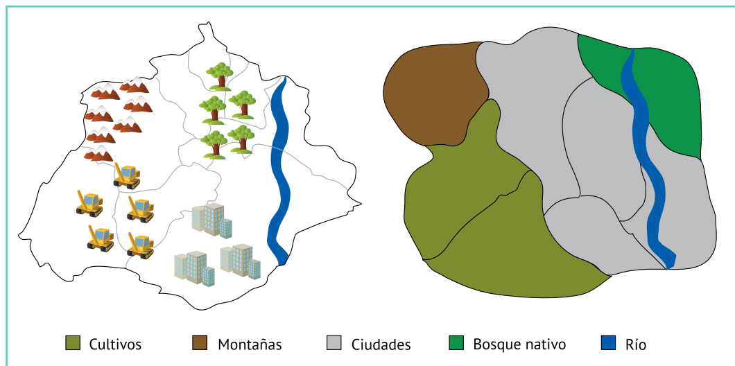
Mapa 1. Municipio de Climatito: geografía física.
