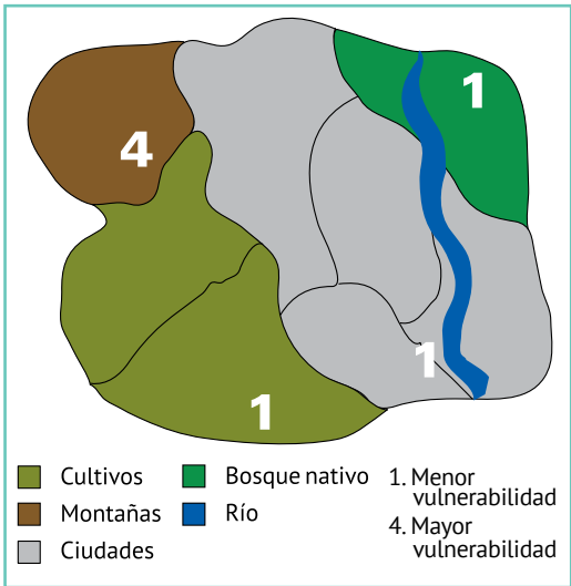
Mapa 7. Municipio de Climatito: grado de vulnerabilidad a sequías
