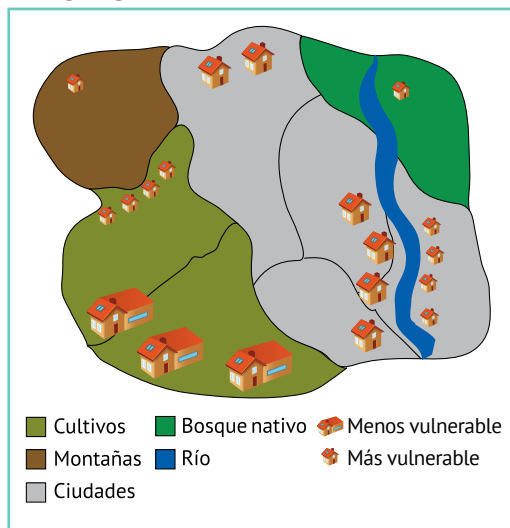
Mapa 6. Municipio de Climatito: grados de vulnerabilidad, según región
