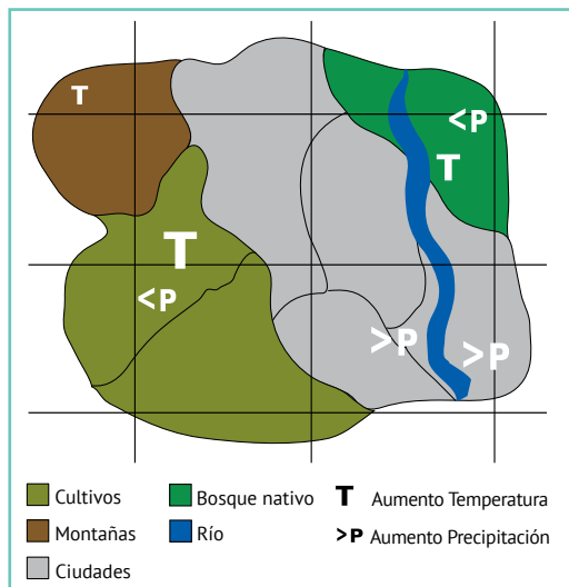
Mapa 3. Municipio de Climatito: escenarios de cambio climático
