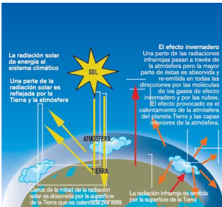
Figura 1. Descripción del Efecto Invernadero
