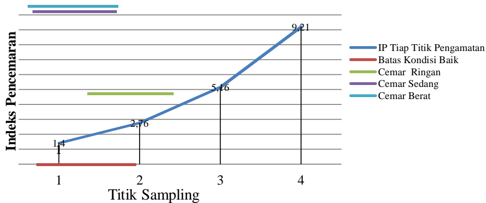
Gambar 4. Grafik indeks pencemaran (IP) Sumber : Hasil Analisis, 2018
