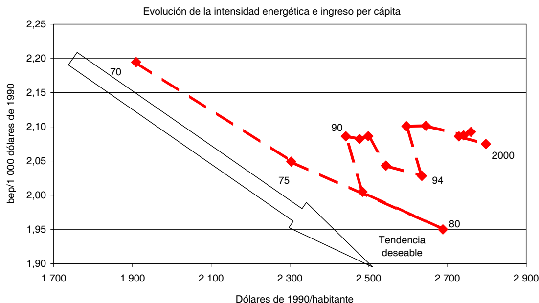
Gráfico VI.4 AMÉRICA LATINA Y EL CARIBE: EVOLUCIÓN DE LA INTENSIDAD ENERGÉTICA E INGRESO PER CÁPITA, 1970-2000
